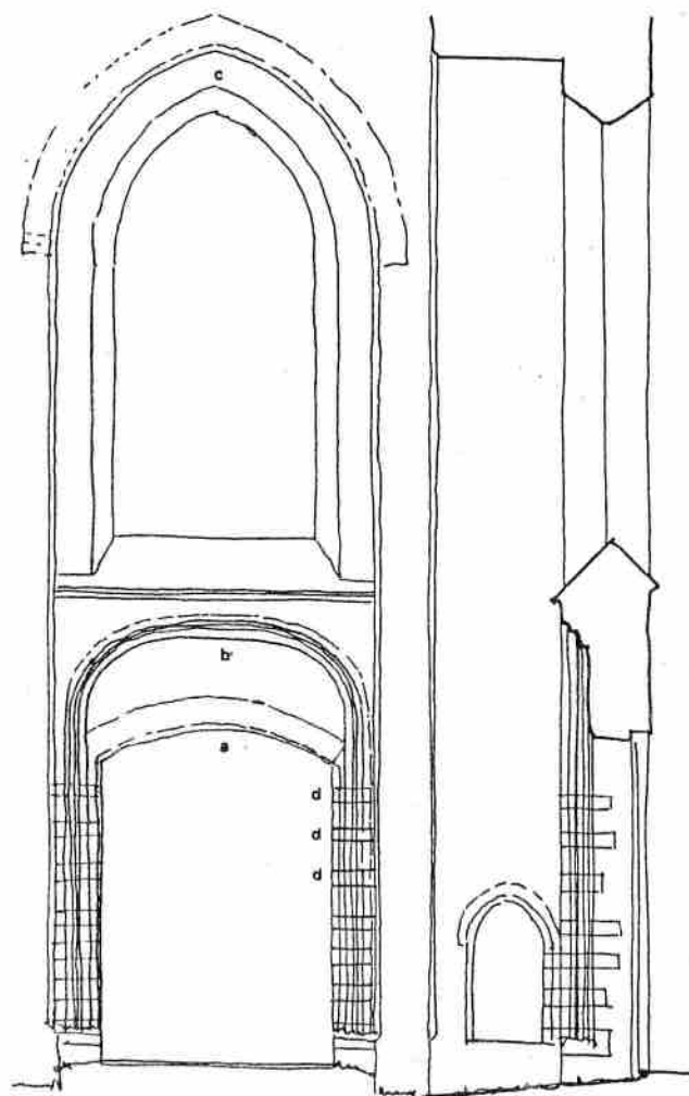
fig. 4 Toreningang aan de westzijde, waarboven lichtvenster voor het kerkportaal. a Segmentboogvormige ingang b Korfboog c Spitsboog d Speklagen van tufsteen
