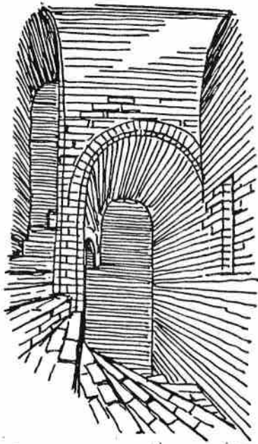
fig. 6 Gemetselde spiltrap in de traptoren, waarboven de vierkante plattegrond van de aanbouw wordt overwelfd met tongewelfjes ter grootte van een kwart van de inwendige maat van de traptoren, die het klimmen van de trap volgen en waarop de bovengelegen treden rusten.
