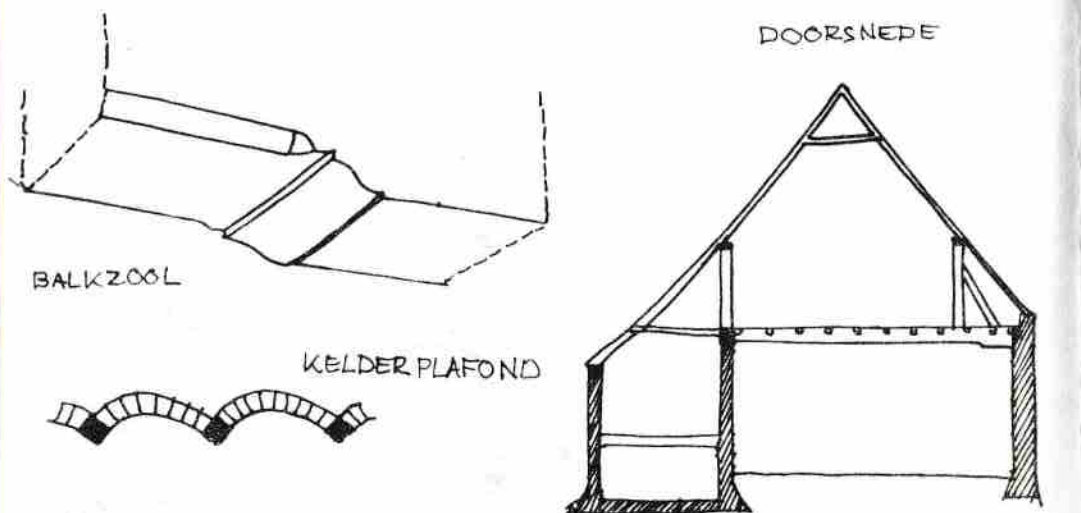
2. Doorsnede en constructiedetails (schetsmatig).
