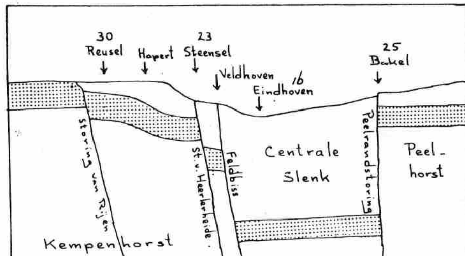
Schematische doorsnede door de Centrale Slenk.
