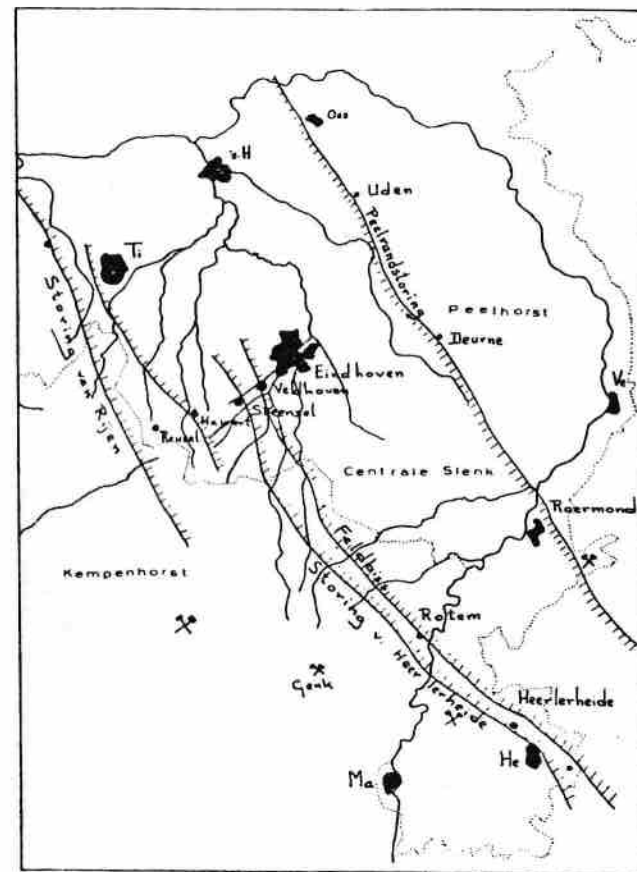
Schematisch overzicht van de storingen in Oost-Brabant en omgeving (naar J. C. van den Toorn, 1962)
